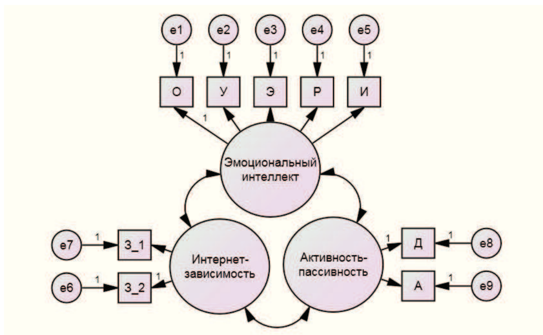
Рис. 11. Модель идентификации
