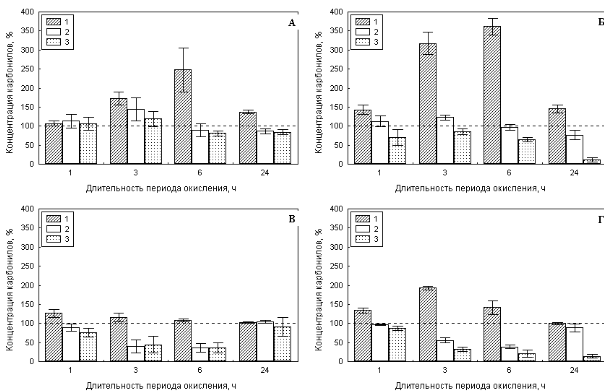
Рис. 6. Влияние буферных растворов (pH 6,0) на основе карбоновых кислот на содержание КС в липосомах. Окисление инициировали 2,5 мМ \text{CuSO}_4 (А, Б) или \text{Cu}(\text{CH}_3\text{COO})_2 (В, Г) в присутствии 0,8 мМ \text{H}_2\text{O}_2 . 1 – ацетатный буфер, 2 – сукцинатный буфер, 3 – цитратный буфер. Концентрация буферообразующих веществ 2 мМ (А, В) и 10 мМ (Б, Г). За 100 % принимали содержание карбонильных соединений в липосомах после соответствующего периода окисления в отсутствие карбоновых кислот (пунктирная линия). Усреднение результатов 4 экспериментов.
