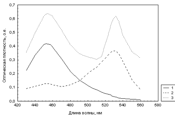
Рис. 2. Спектры поглощения веществ, образующихся при взаимодействии ТБК, продуктов ПОЛ фосфатидилхолиновых липосом (2,38 мг липида/мл суспензии) и сульфата меди (II) в среде трихлоруксусной кислоты (спектры сняты относительно раствора ТБК): 1 – ТБК + 0,625 мМ Cu 2+ ; 2 – ТБК + липосомы после 18-часового автоокисления; 3 – ТБК + липосомы после 18-часового автоокисления + 0,625 мМ Cu 2+ .
