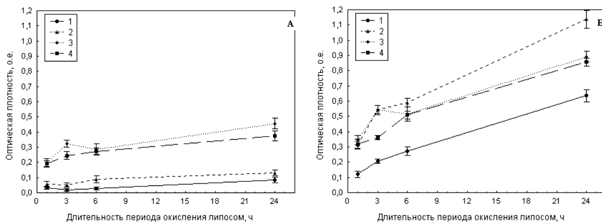
Рис. 1. Поглощение при длинах волн 452 нм (А) и 532 нм (Б) хромогенов, образующихся при взаимодействии карбонильных соединений суспензии липосом (2,38 мг липида/мл суспензии), подвергнутых автоокислению при 37 °С, и ТБК в среде трихлоруксусной кислоты: 1 – в отсутствие катионов металлов; 2 – в присутствии 0,625 мМ Fe 2+ ; 3 – в присутствии 0,625 мМ Cu 2+ ; 4 – в присутствии 0,625 мМ Fe 2+ и 0,625 мМ Cu 2+ . Усреднение результатов 4 экспериментов.
