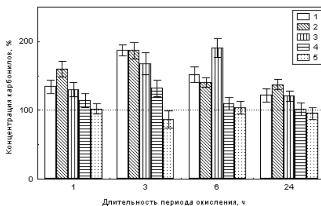
Рис. 5. Влияние 20 мМ MES–NaOH буферного раствора (pH 6,8) на содержание карбонильных соединений в липосомах в ходе автоокисления (1) и окисления, индуцированного: 2,5 мМ \text{CuSO}_4 (2), 2,5 мМ \text{CuSO}_4 + 0,8 мМ \text{H}_2\text{O}_2 (3), 2,5 мМ \text{Cu}(\text{CH}_3\text{COO})_2 (4), 2,5 мМ \text{Cu}(\text{CH}_3\text{COO})_2 + 0,8 мМ \text{H}_2\text{O}_2 (5). За 100 % принимали значение показателя на соответствующий момент времени в контрольном незабуференном препарате липосом. Усреднение результатов 4 экспериментов.
