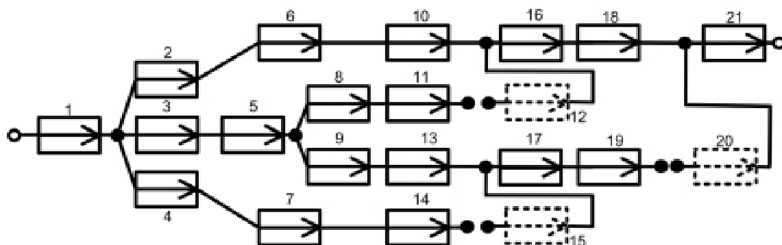
Рис. 3 - Узловая модель исследуемой сети
