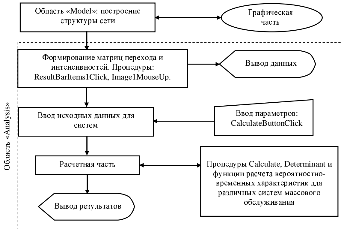
Рисунок 2 – Укрупненный алгоритм работы программы
