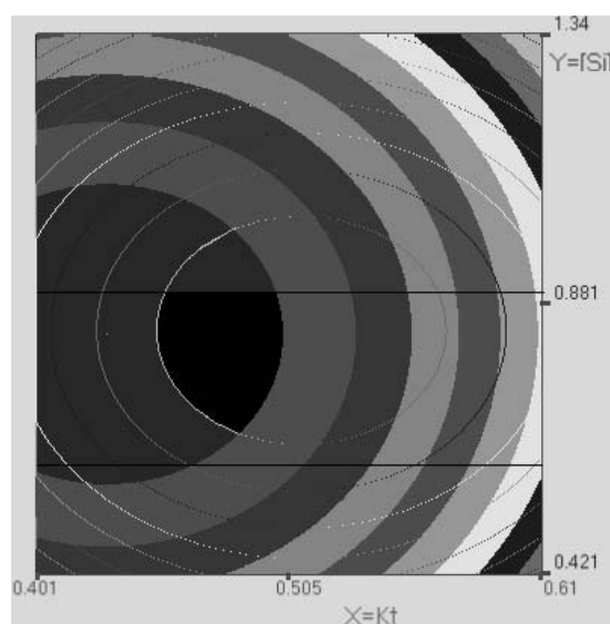
Рис. 2. Трехмерная диаграмма для определения оптимальных значений критерия оценки теплового состояния, соответствующих максимальной производительности печи и минимальному расходу суммарного топлива
